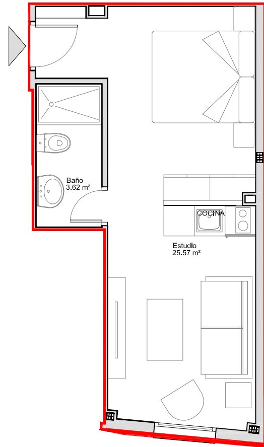
Apartamento 5 · Planta primera
